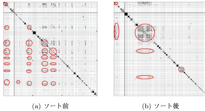
図 6: 年度区切り散布図 (Parser)
