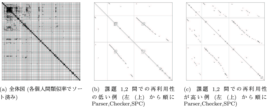
図 7: 個人区切り散布図 (Parser+Checker+SPC)
