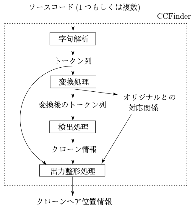
図 1: CCFinder の処理手順
